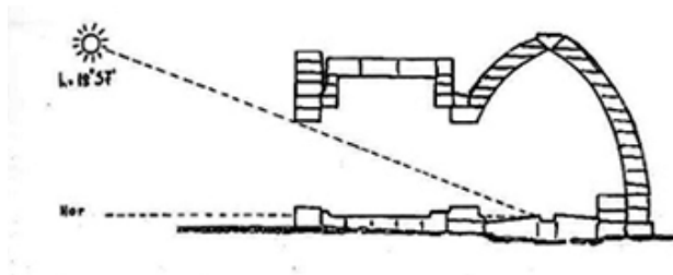
Обр. 5. Вертикален разрез през тракийска култова сграда под могила Голяма Арсеналка, от [16: 166] по Stoev, Stoeva 2006
