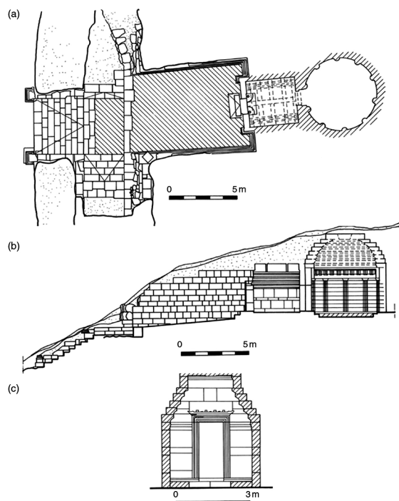
Обр. 6. Хоризонтален план и надлъжен вертикален разрез на храма под „Четиньова могила“, с. Старосел, община Хисаря (Stoyanova, D. Tomb Architecture. – In: Valeva, J., E. Nankov, D. Graninger. A Companion to Ancient Thrace. Oxford: Oxford University Press, 2015, p. 162)
